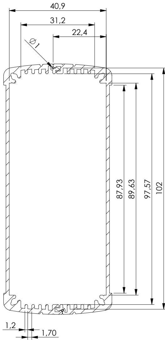
SEZIONE A-A
